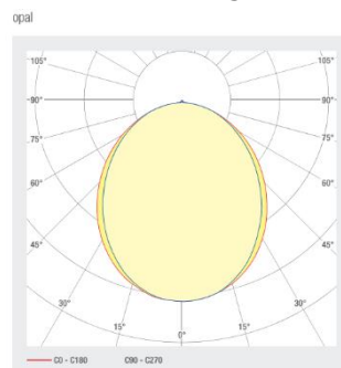
Abstrahlungen
