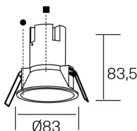
Ausschnitt Ø 75mm
