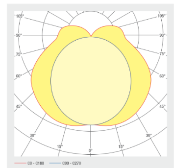
Abstrahlung
