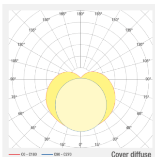
Abstrahlung Diffus
