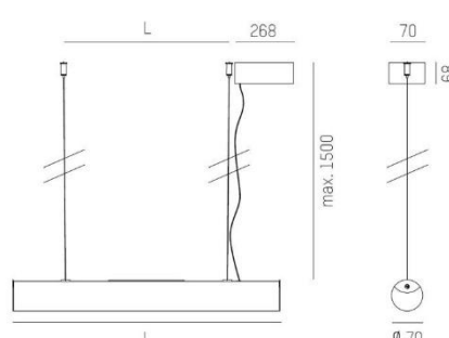
VALO PDI Massskizze 2266 – 3386mm
