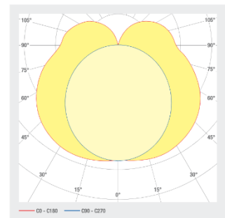
Abstrahlung
