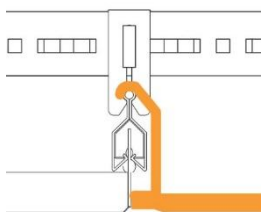
Befestigungsfeder Gema-Armstrong Q-Clip
