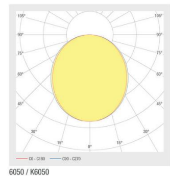
Abstrahlung
