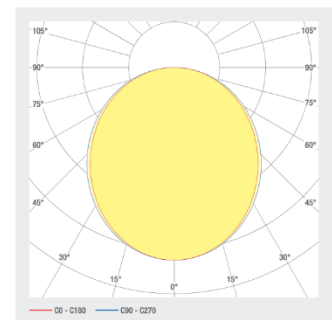
Abstrahlung
