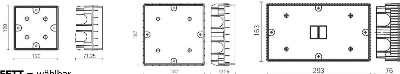
STAMP Einbaugehäuse & Masse
