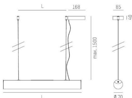
VALO PDI Massskizze 586 – 1706mm
