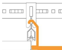
Befestigungsbügel Gema-Armstrong UK mit H28 Profil
