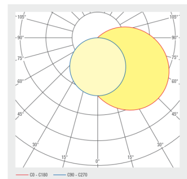
Abstrahlung
