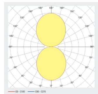
Abstrahlung
