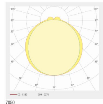
Abstrahlung
