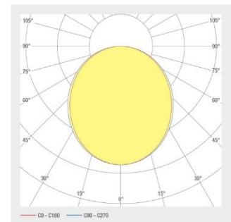
Abstrahlung
