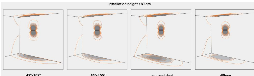
Optiken
