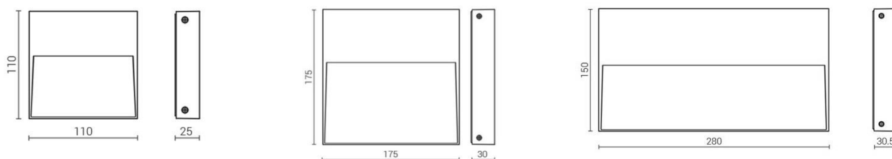
STAMP Einbaugehäuse & Masse
