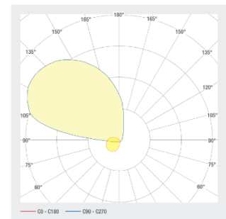
Abstrahlung
