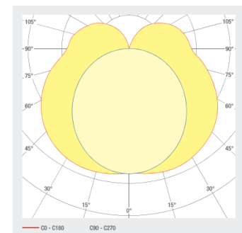
Abstrahlung
