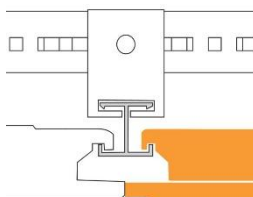
Befestigungsbügel Gema-Armstrong UK mit H28 Profil
