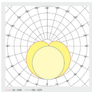
Abstrahlung Diffus
