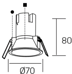
Ausschnitt Ø 62mm
